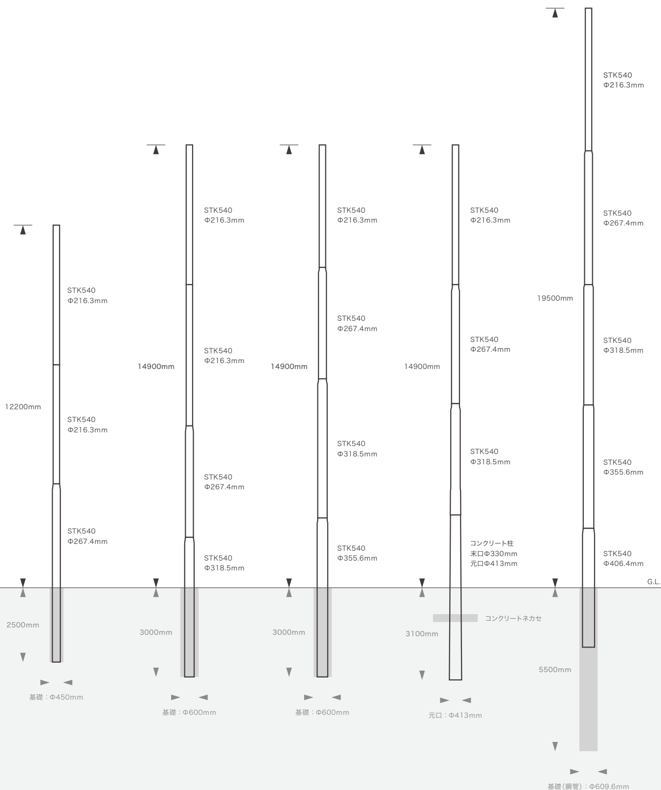
地上高さ 12m 品番：YSJ・K-12 ジョイマスト
