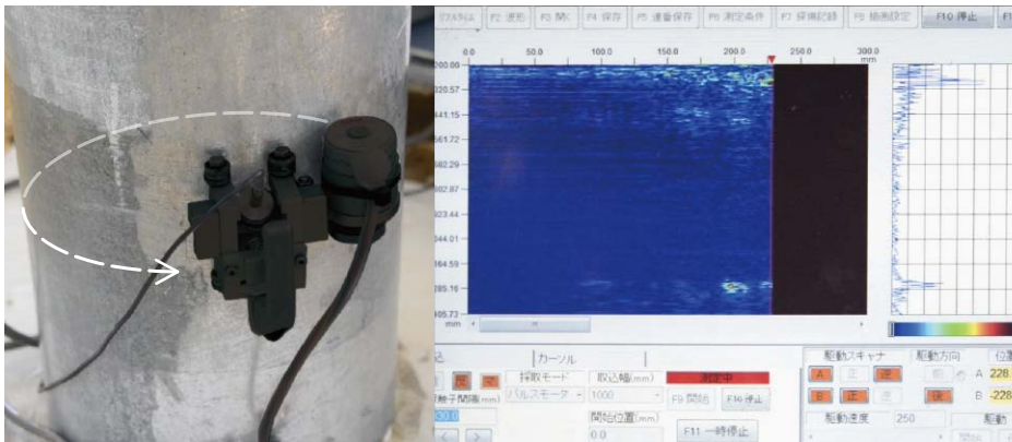
自走式センサーからのスクリーニング情報を端末へ送信、展開図画像により鋼管の腐食状況を確認できます。
